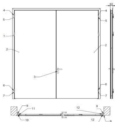
Рис. 1 Ворота металлические двупольные
